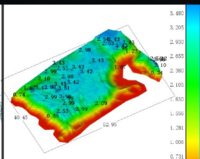
堆体测量
